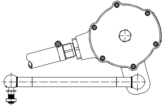
Bras de couple assurré par une barre à tête sphérique
