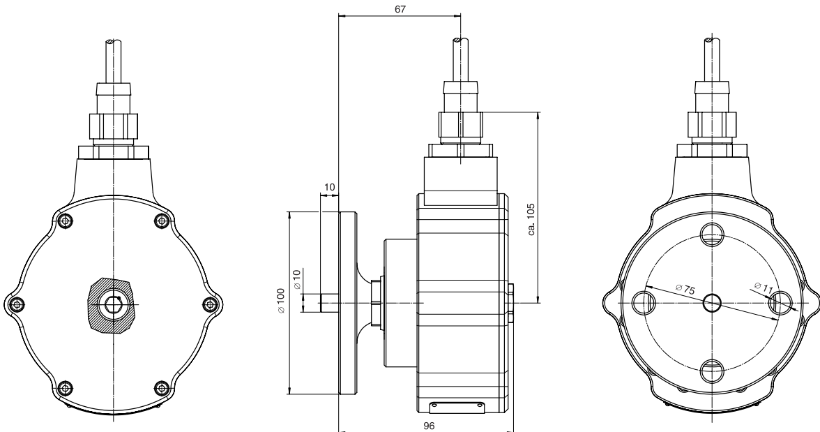
Dimensions du GEL 2701 (avec bride mobile RF 1)
